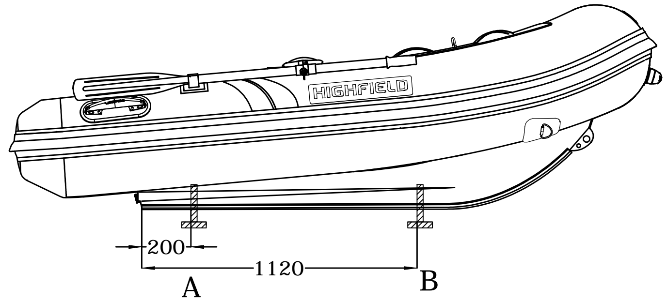
LONGITUDINAL PROFILE
